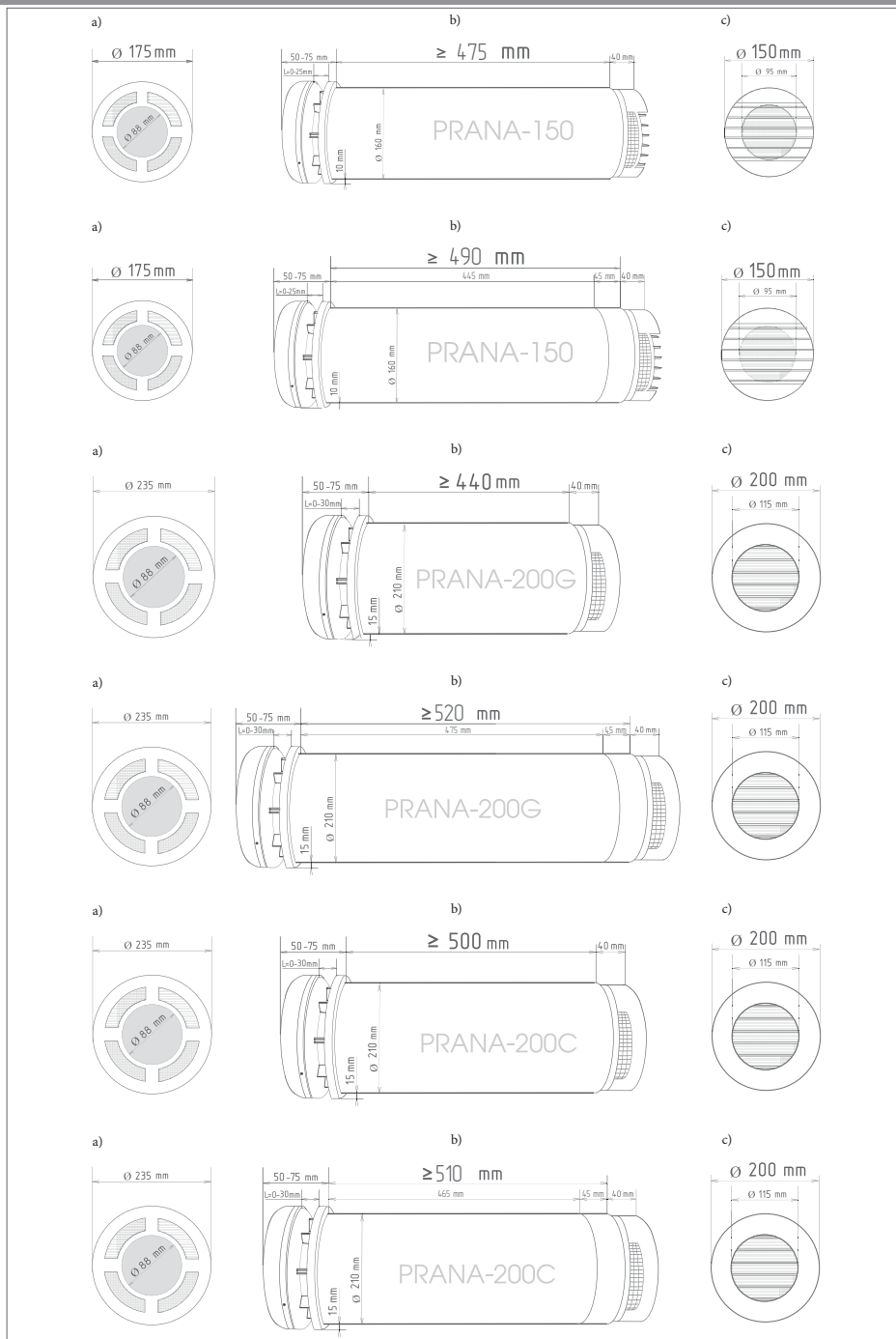
Rys. 3 Wymiary systemu wentylacyjnego «PRANA-150 Premium Plus», «PRANA-200G Premium Plus», «PRANA-200C Premium Plus»:
